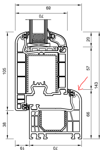
Utåtgående dörr
